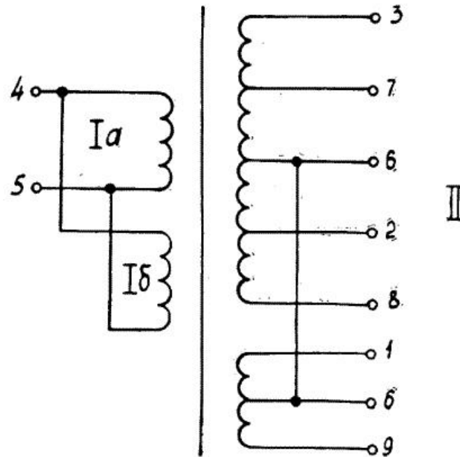
Рис. 2. Схема электрическая принципиальная и намоточные данные трансформатора ТВВТ-9
