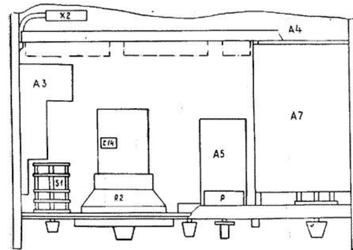
Рис. 1. Вид сверху
