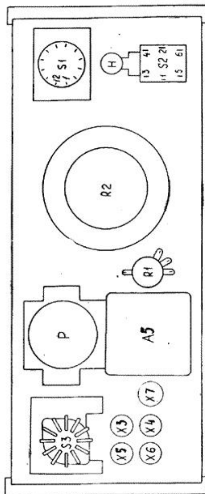
Рис. 2. Вид на переднюю панель
