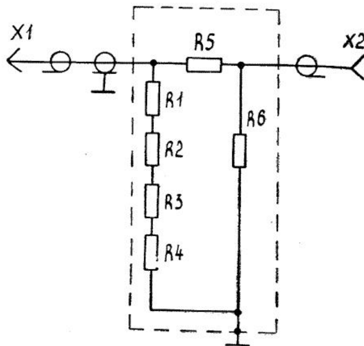
СХЕМА ЭЛЕКТРИЧЕСКАЯ ПРИНЦИПИАЛЬНАЯ ВНЕШНЕГО АТТЕНЮАТОРА, 40 дБ
