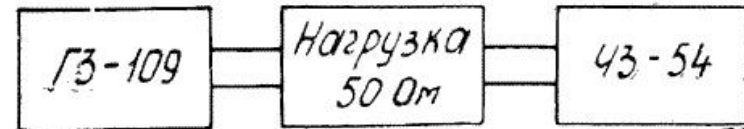
Рис. 2. Схема структурная соединения приборов для определения погрешности установки частоты генератора по шкале частот
