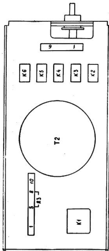
Рис. 6. Схема электрическая расположения элементов блока трансформаторов (вид снизу)
