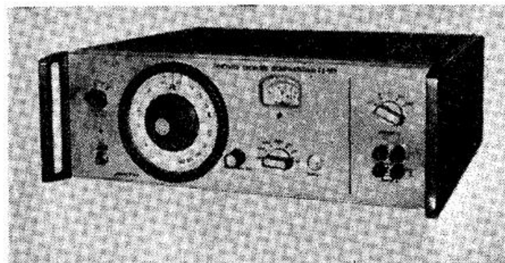
Внешний вид генератора ГЗ-109
