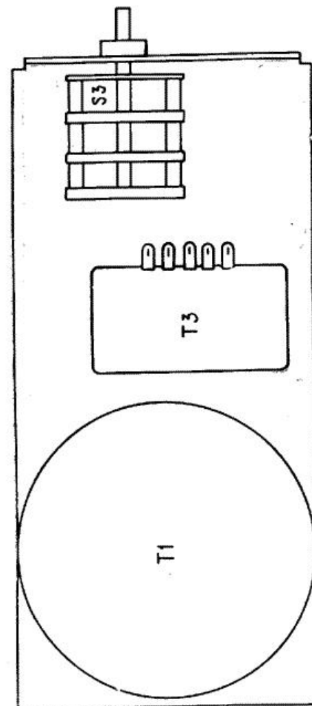
Рис. 5. Схема электрическая расположения элементов блока трансформаторов (вид сверху)
