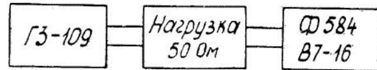
Рис. 3. Схема структурная соединения приборов для определения погрешности установки выходного напряжения генератора
