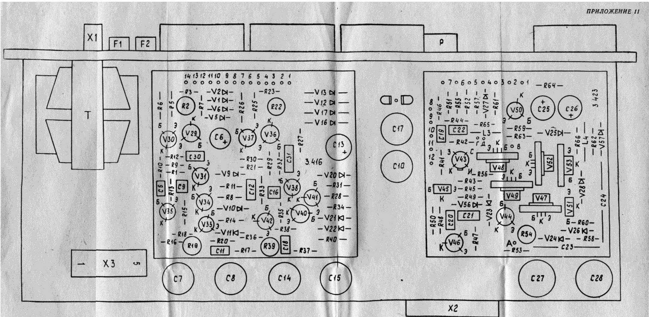
Рис. 7. Схема электрическая расположения элементов блока питания (вид сверху) генератора ГЗ-109
