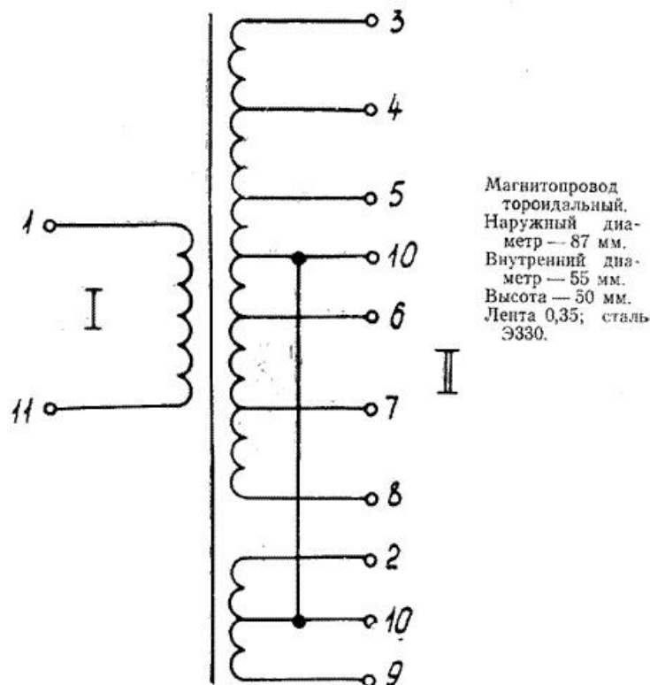
Рис. 1. Схема электрическая принципиальная и на- моточные данные трансформатора ТВТ-43
