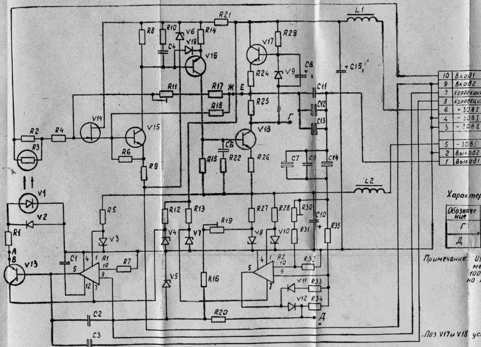
СХЕМА ЭЛЕКТРИЧЕСКАЯ ПРИНЦИПАЛЬНАЯ УСИЛИТЕЛЯ ПРЕДВАРИТЕЛЬНОГО ГЕНЕРАТОРА ГЗ-109
