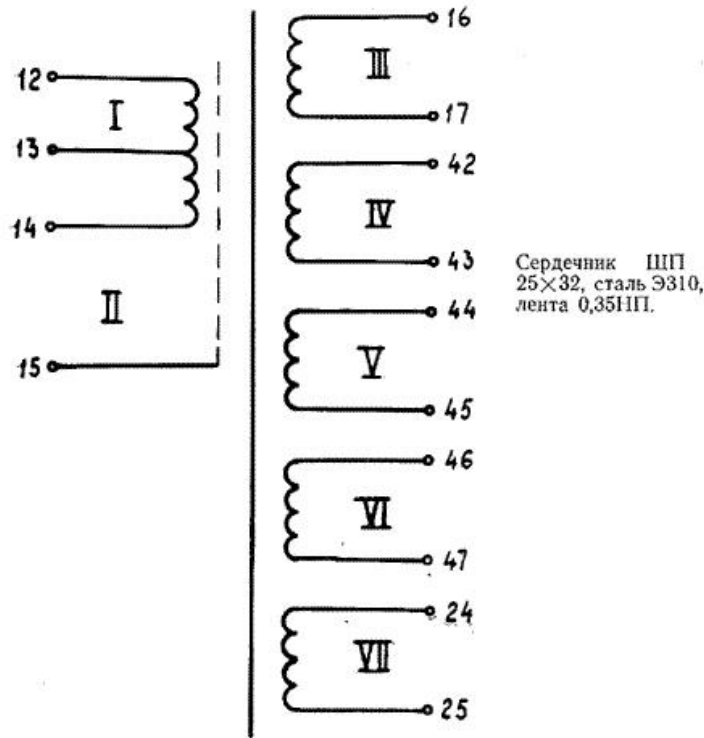
Рис. 5. Схема электрическая принципиальная и намоточные данные трансформатора ТС-16
