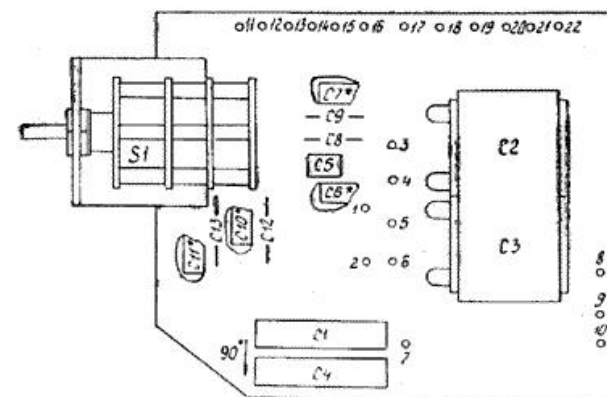
Рис. 3. Схема электрическая расположения элементов блока фазирования
