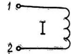
Рис. 4. Схема электрическая принципиальная и намоточные данные индуктивности 330 мкГ
