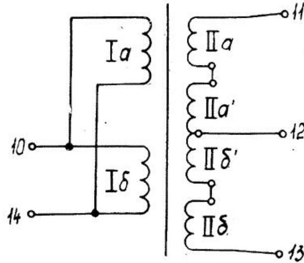
Рис. 3. Схема электрическая принципиальная и намоточные данные трансформатора ТВВТ-8
