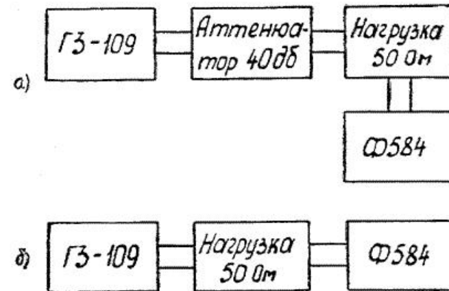
Рис. 4. Схема структурная соединения приборов для определения погрешности ослабления: внешнего аттенюатора 40 дБ (рис. 4, а), встроенного аттенюатора (рис. 4, б)
