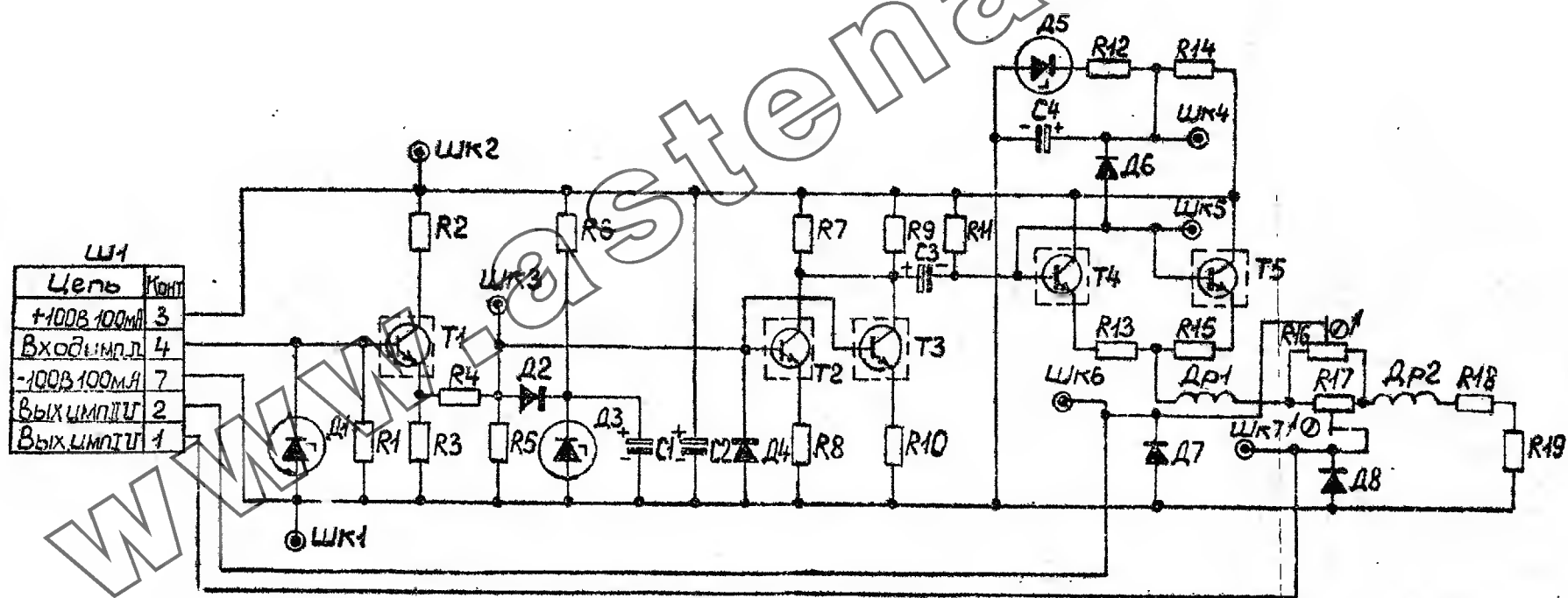
Рис. 7. Модулятор 2.081.320.93.
