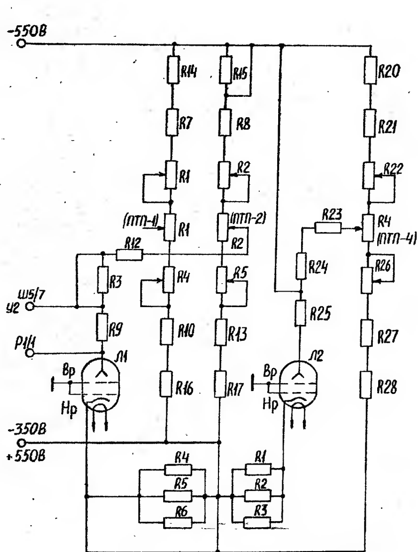
Рис.7 Схема подачи напряжений на клистроны при работе прибора в диапазоне частот 12,7-17,85 ГГц. Обозначение элементов соответствует схеме электрической принципиальной блока высокой частоты (см. рис. 2 приложения).
