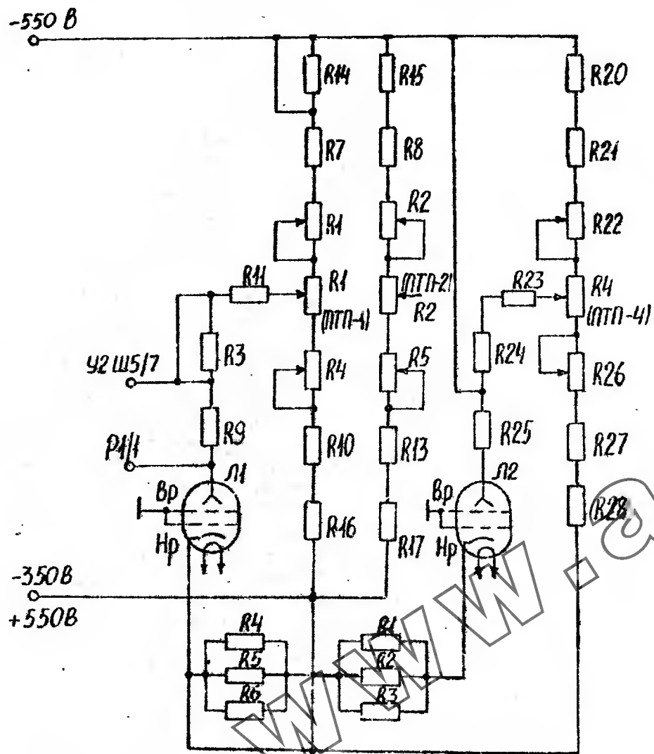
Рис.5. Схема подачи напряжений на клистроны при работе прибора в диапазоне частот 6-9 ГГц.
