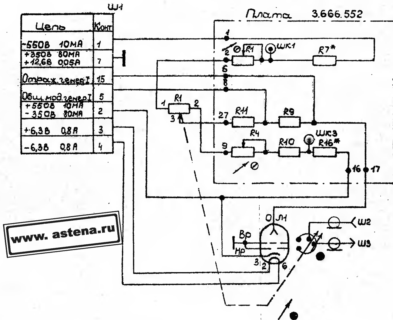
Рис. 5. Блок высокой частоты 6-9 ГГц. Схема электрическая принципиальная 3.269.28133
