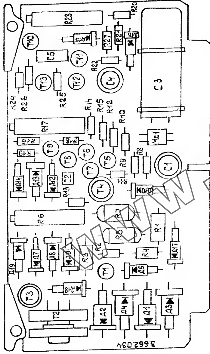
Рис.25. План размещения элементов на плате 3662.034 / Блок питания
