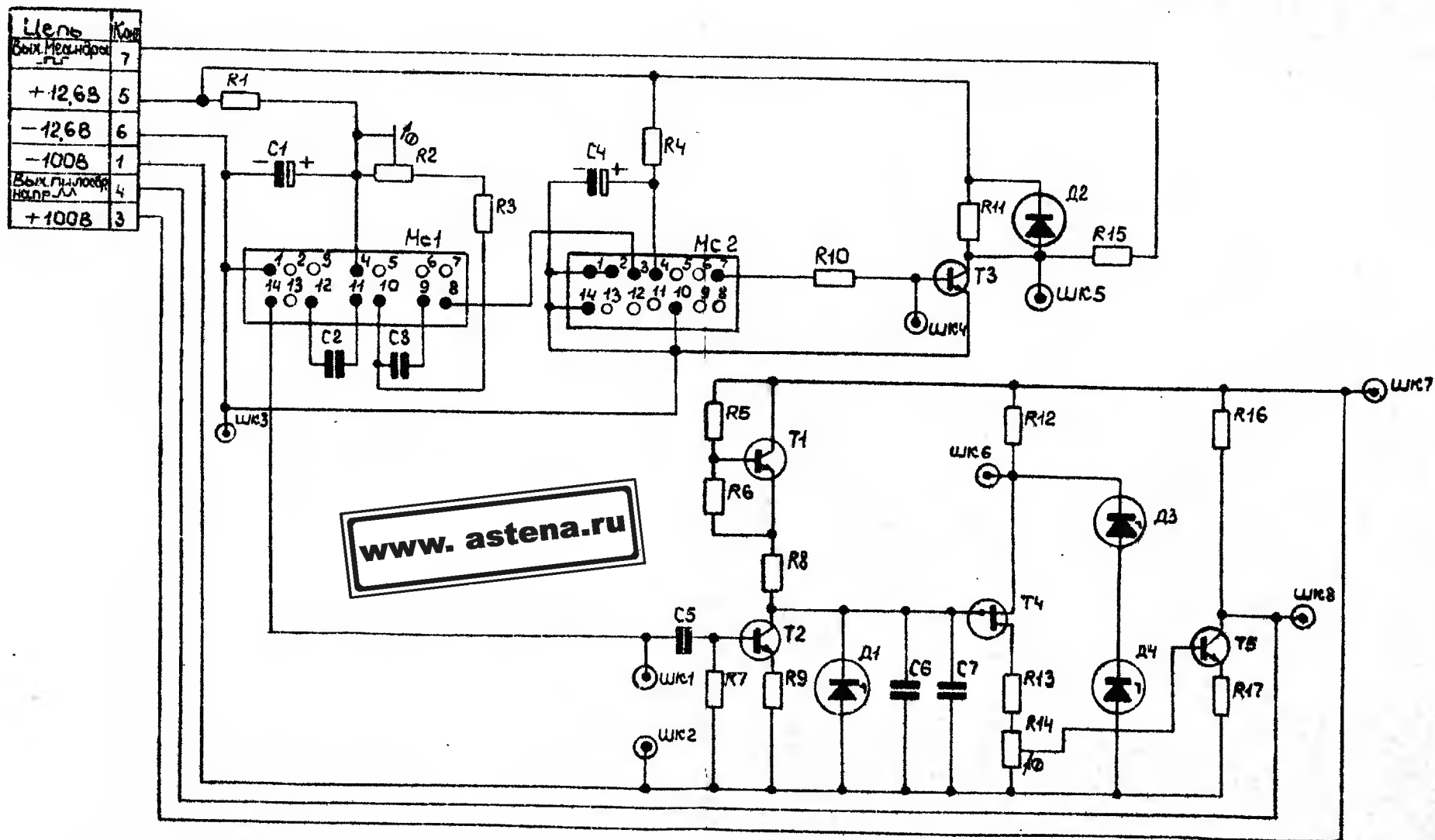
Рис.8. Генераторы меандра и пилообразного напряжения. Схема электрическая принципиальная 3.263.022.93
