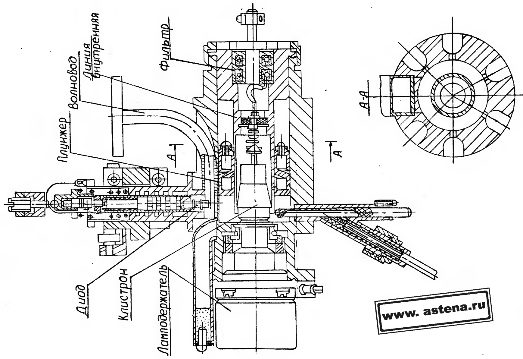
Рис. 10 Гетеродин на диапазон частот 6-9 ГГц
