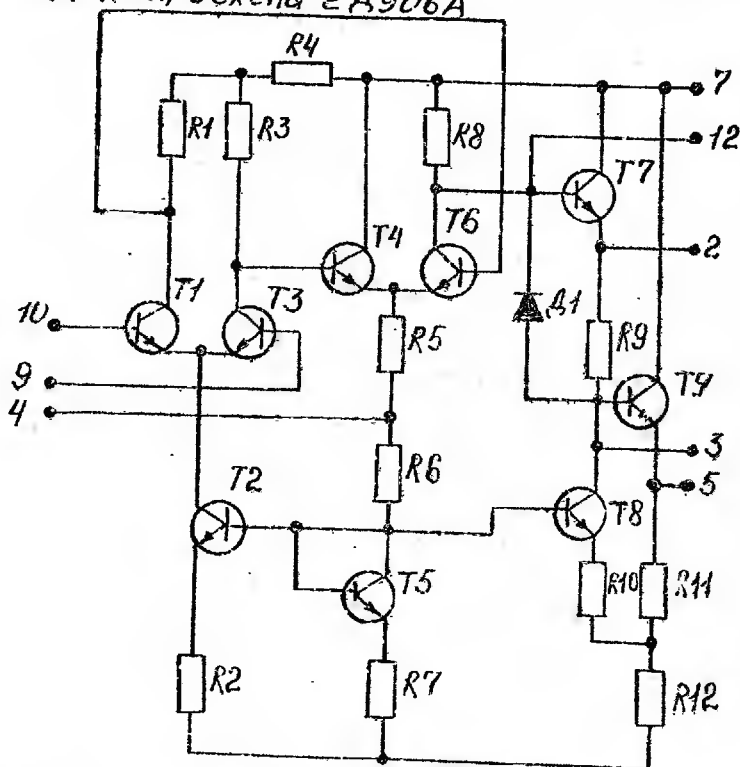
Рис.14. Схема электрическая принципиальная микросхемы 140УД1А
