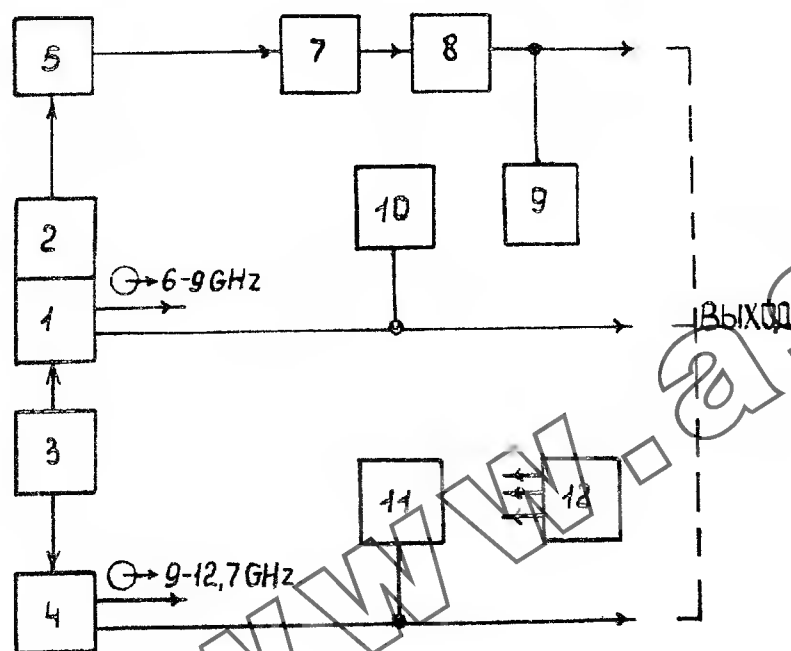
Рис.2. Схема структурная электрическая генератора ГЧ-111
