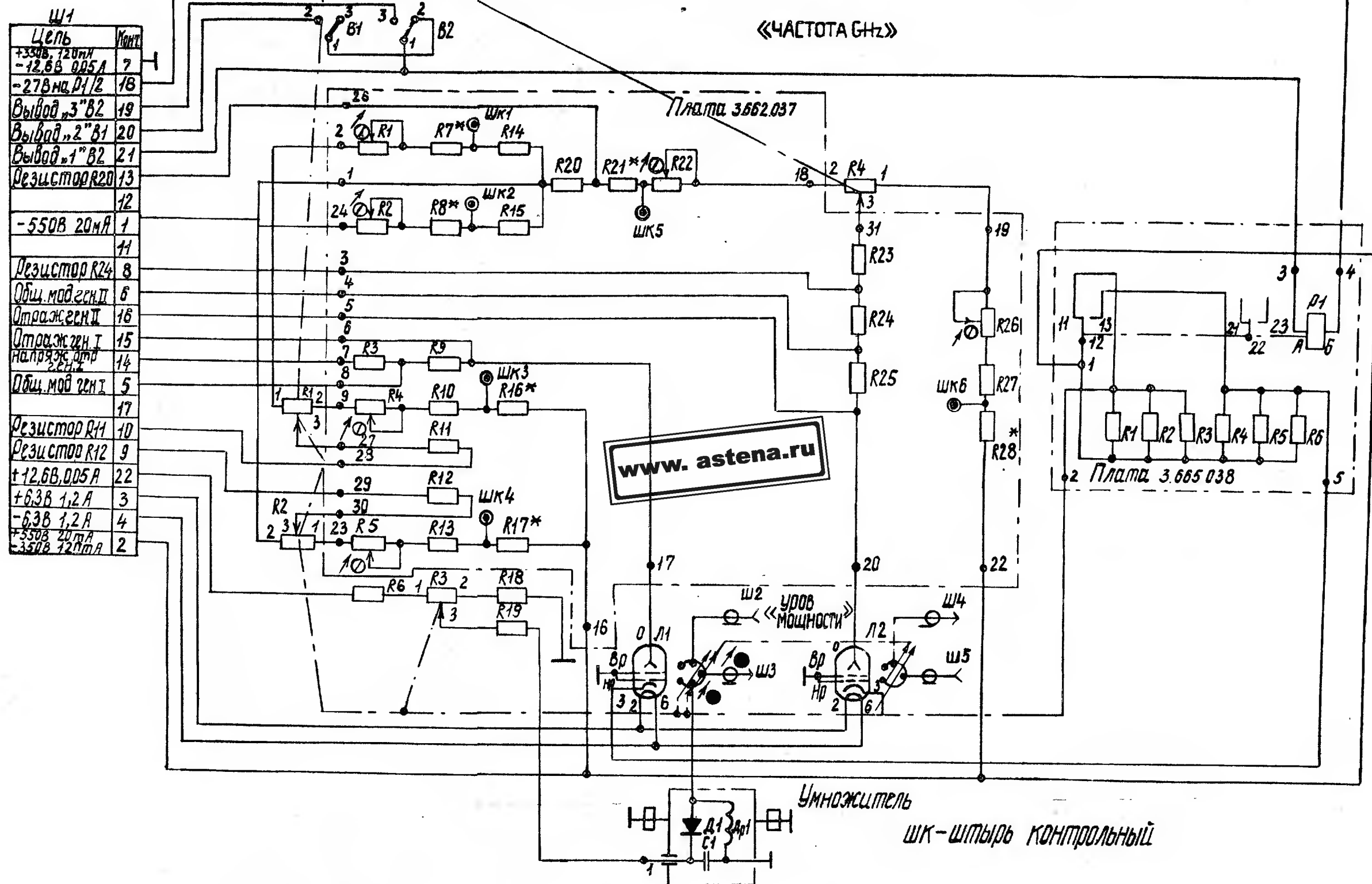
Рис. 4 Блок высокой частоты. Схема электрическая принципиальная 3.269.24833
