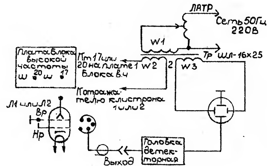
Рис. 14. Схема для регулировки автогенераторов после смены клистрона
