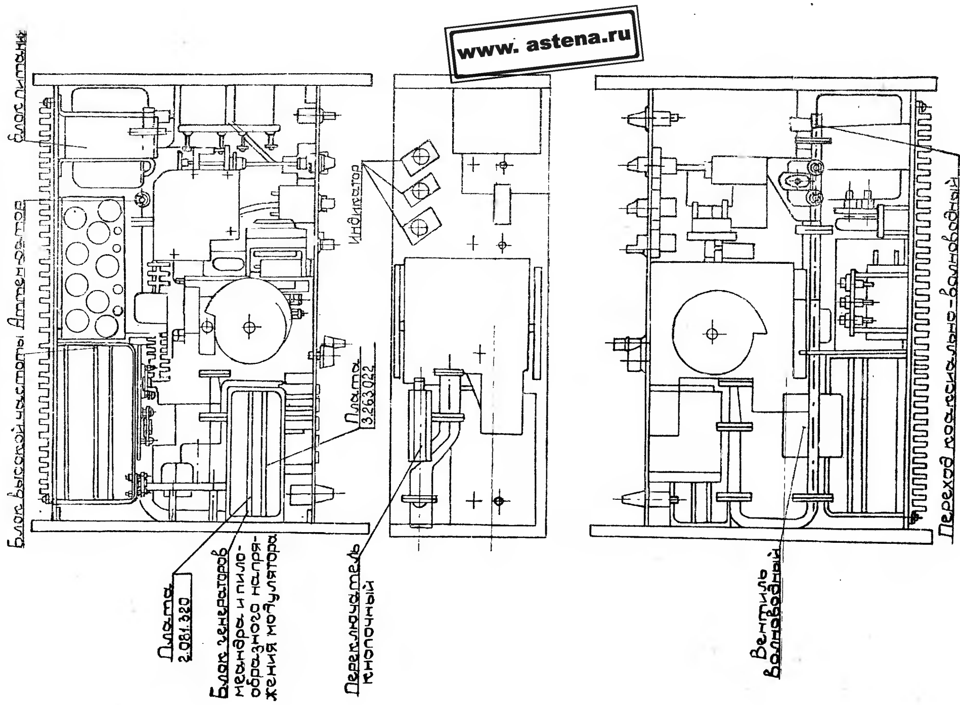
Рис.15. План размещения узлов генератора сигналов высокочастотного ГЧ-ММ
