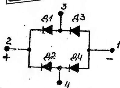
Рис.13 Схема электрическая принципиальная микросхемы 2А906А
