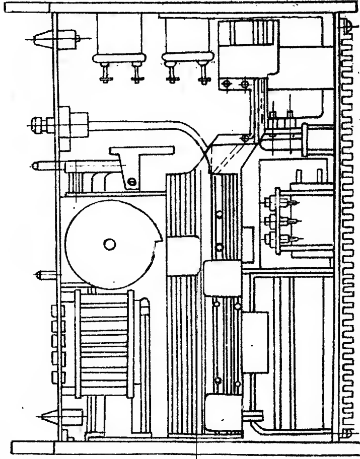
Рис.16. План размещения узлов генераторов сигналов высокочастотных ГЧ-111/6
