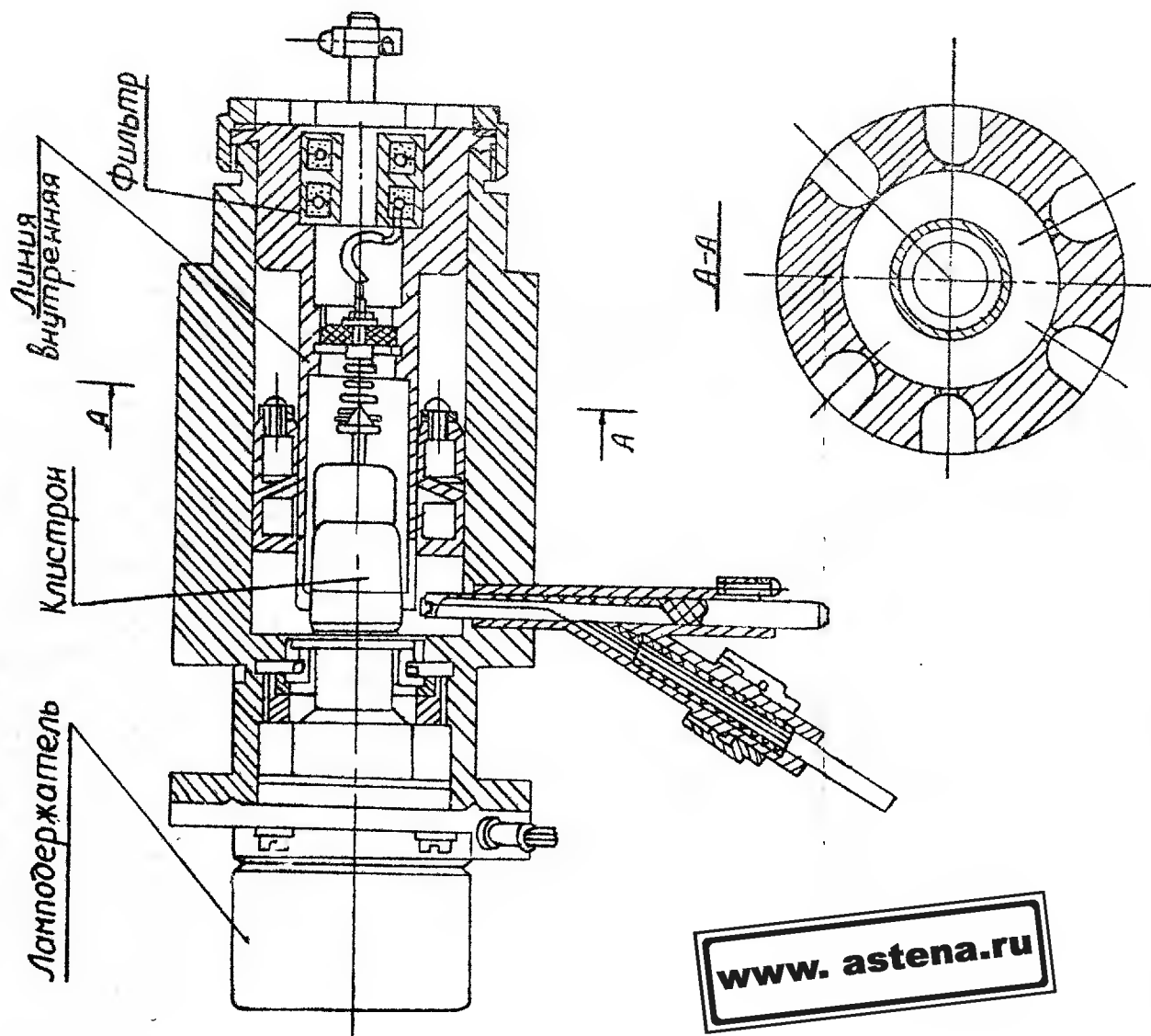
Рис.13. Гетеродин на диапазон частот 6-9 ГГц генератора ГЧ-ИИ/а
