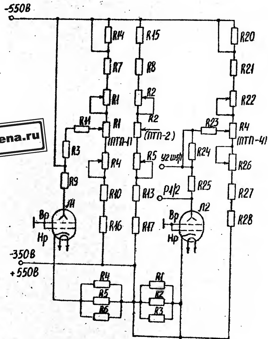
Рис.6 Схема подачи напряжений на клистроны при работе прибора в диапазоне частоты 9-12,7 ГГц. Обозначение элементов соответствует схеме электрической принципиальной блока высокой частоты (см. рис. 2 приложения).
