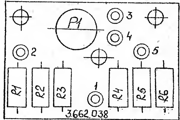
Рис. 17. План размещения элементов на платах блока высокой частоты генератора Г4-111.
