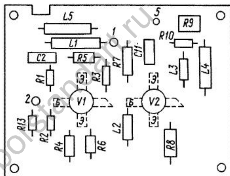
Рис. 3. Усилитель ВЧ 2.030.055
