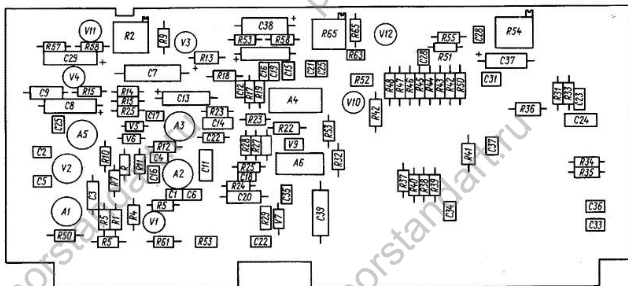
Рис. 4. Усилитель постоянного тока 2.032.027 (вид со стороны монтажа)
