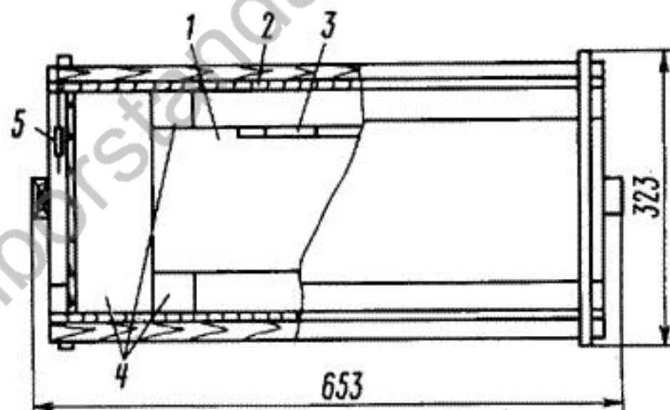
Рис. 9. Схема упаковки:
