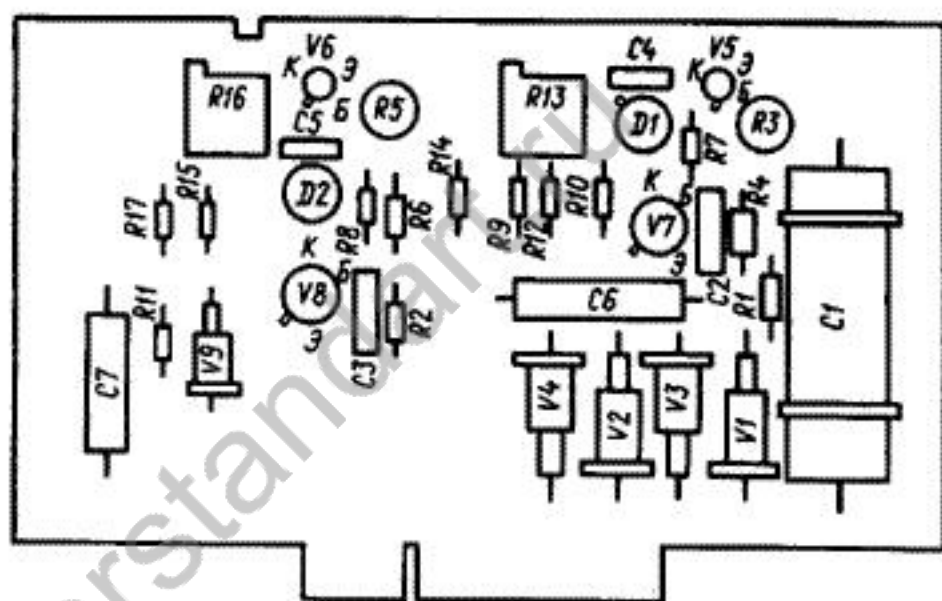
Рис. 18. Блок стабилизаторов напряжения 3.233.120
