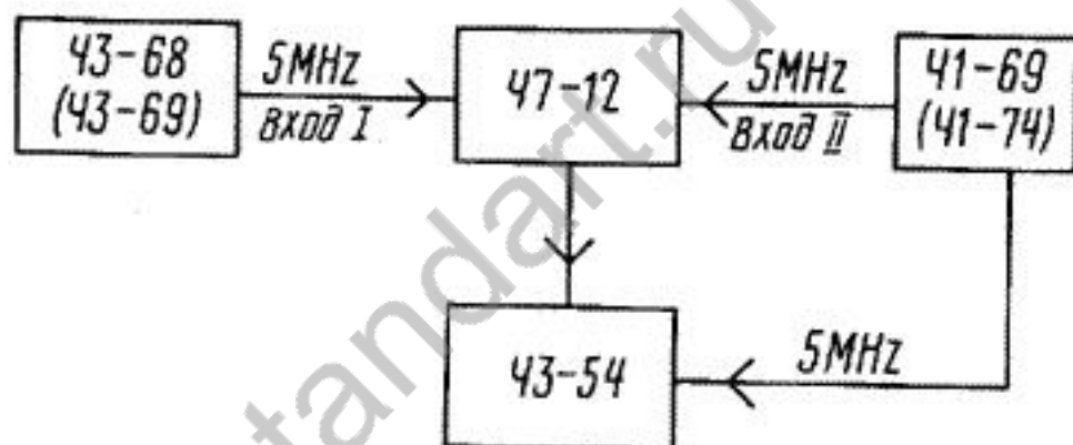
Рис. 8. Структурная схема измерения частоты кварцевого генератора
