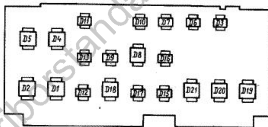
Рис. 8. Устройство вычислительное управляющее 3.035.033 (вид со стороны микросхем)
