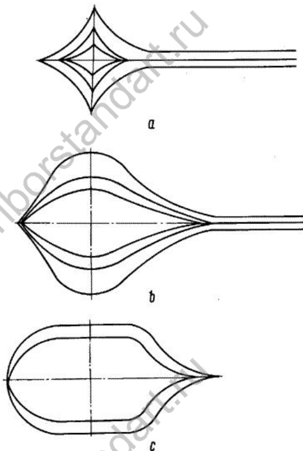
Рис. 7. Осциллограммы нулевых биений:
