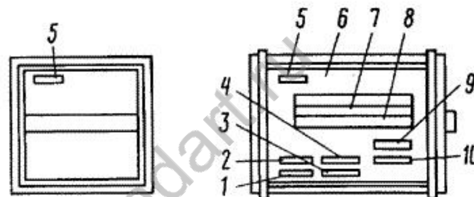
Рис. 10. Расположение маркировки:
