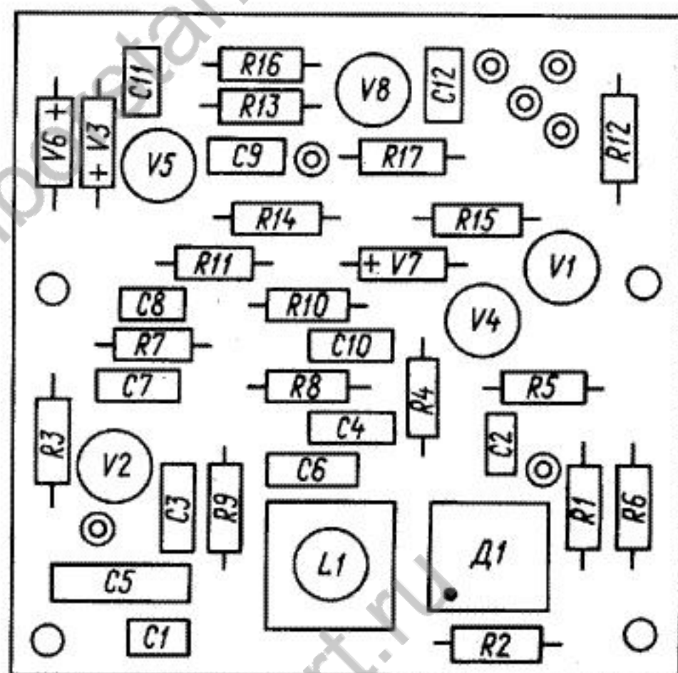
Рис. 19. Генератор кварцевый 3.261.006
