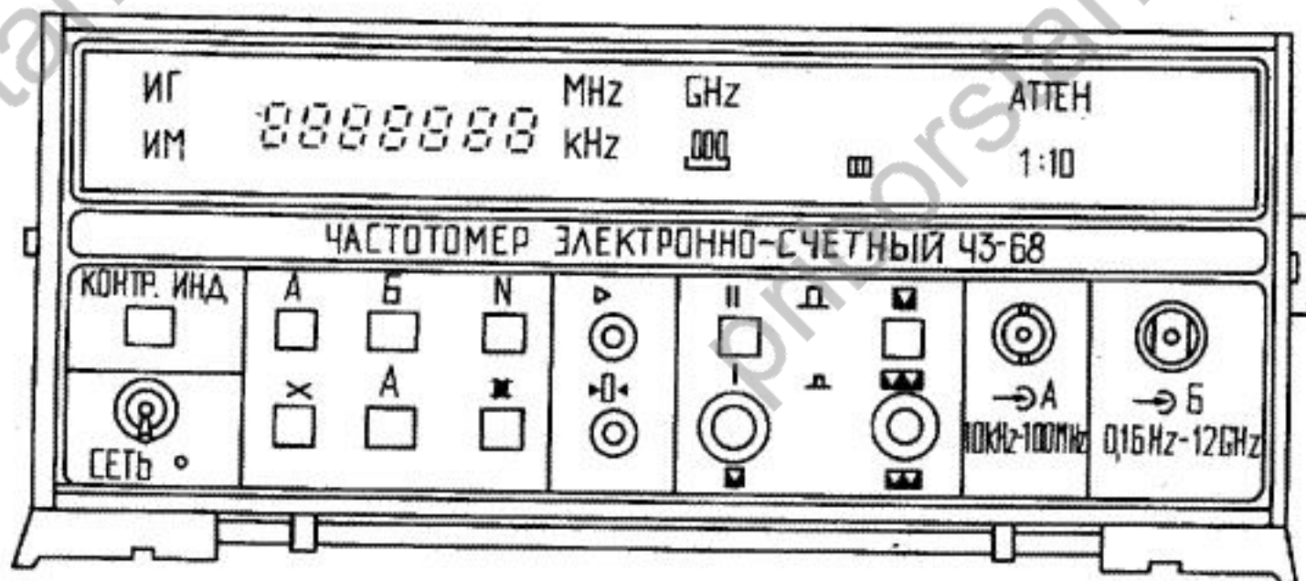
Рис. 1. Частотомер ЧЗ-68
