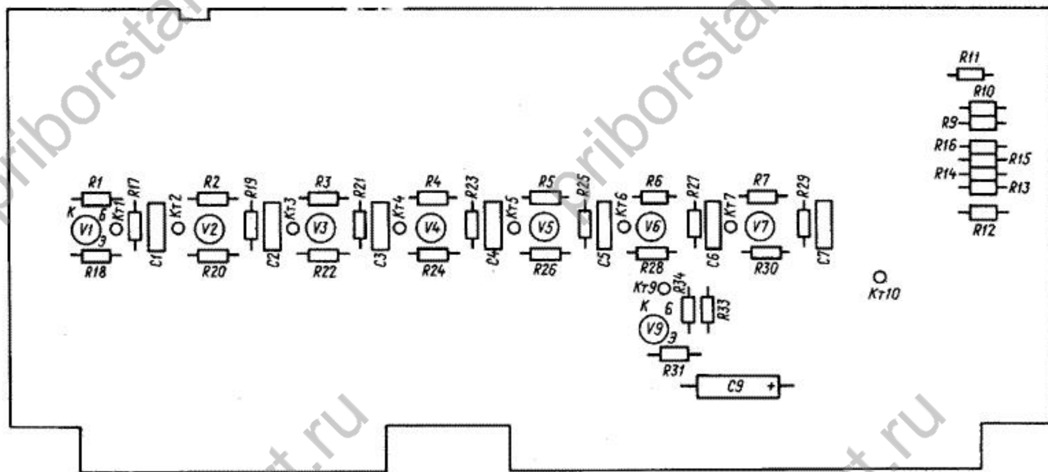
Рис. 14. Устройство запоминающее программируемое 3.065.066 (вид со стороны монтажа)
