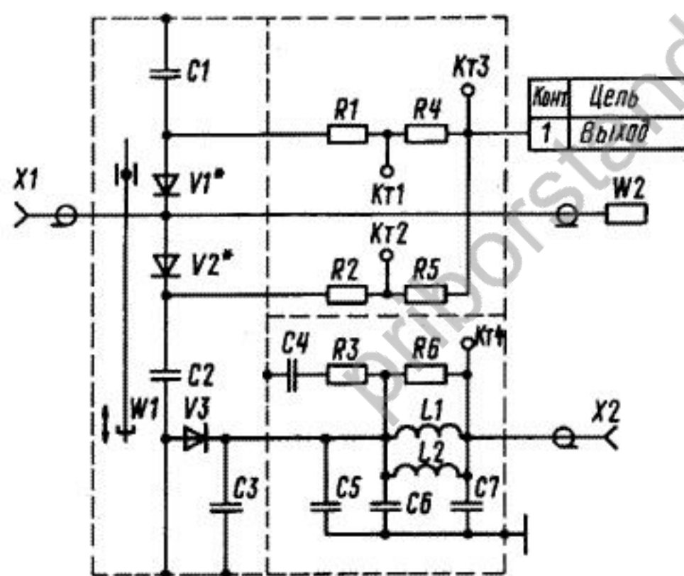
Рис. 14. Схема электрическая принципиальная смесителя СВЧ 2.245.013
