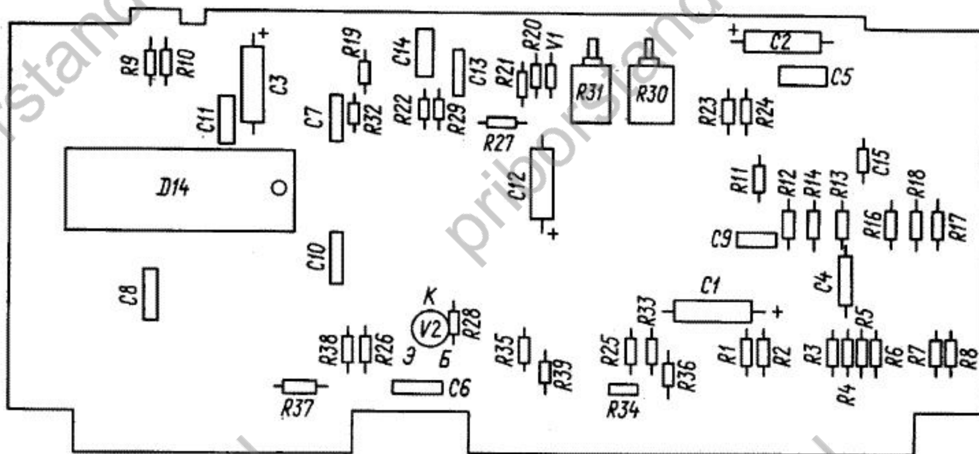
Рис. 7. Устройство вычислительное управляющее 3.035.033 (вид со стороны монтажа)
