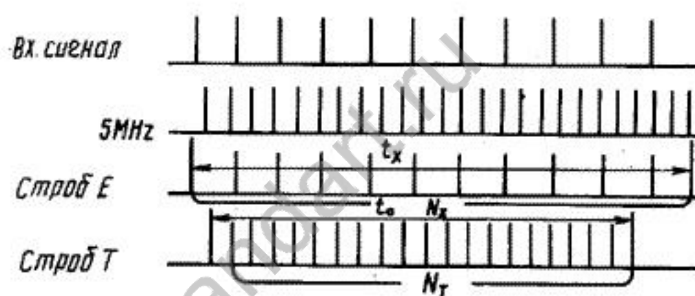
Рис. 3. Формирование измеряемого интервала времени
