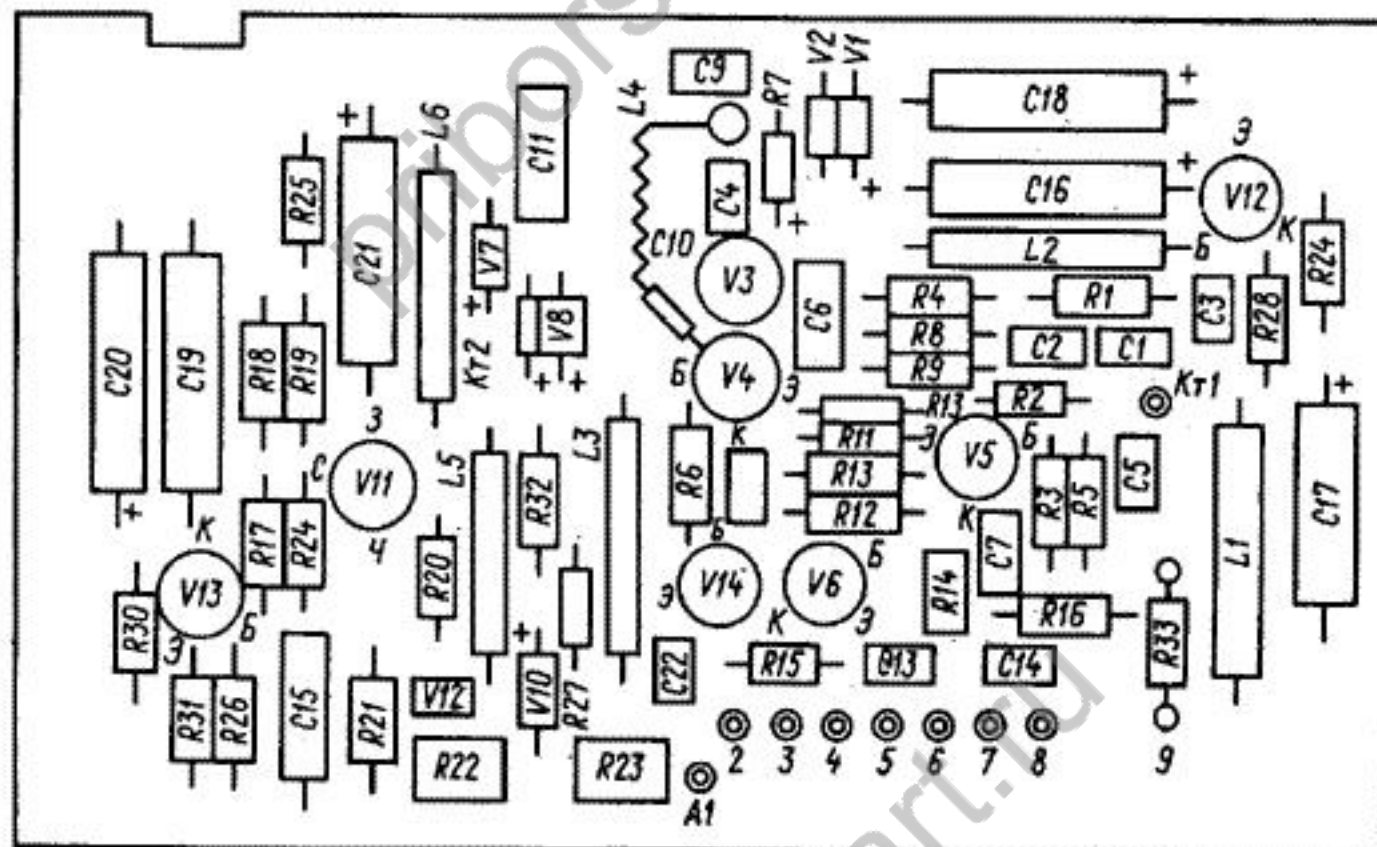
Рис. 6. Гетеродин 2.205.017
