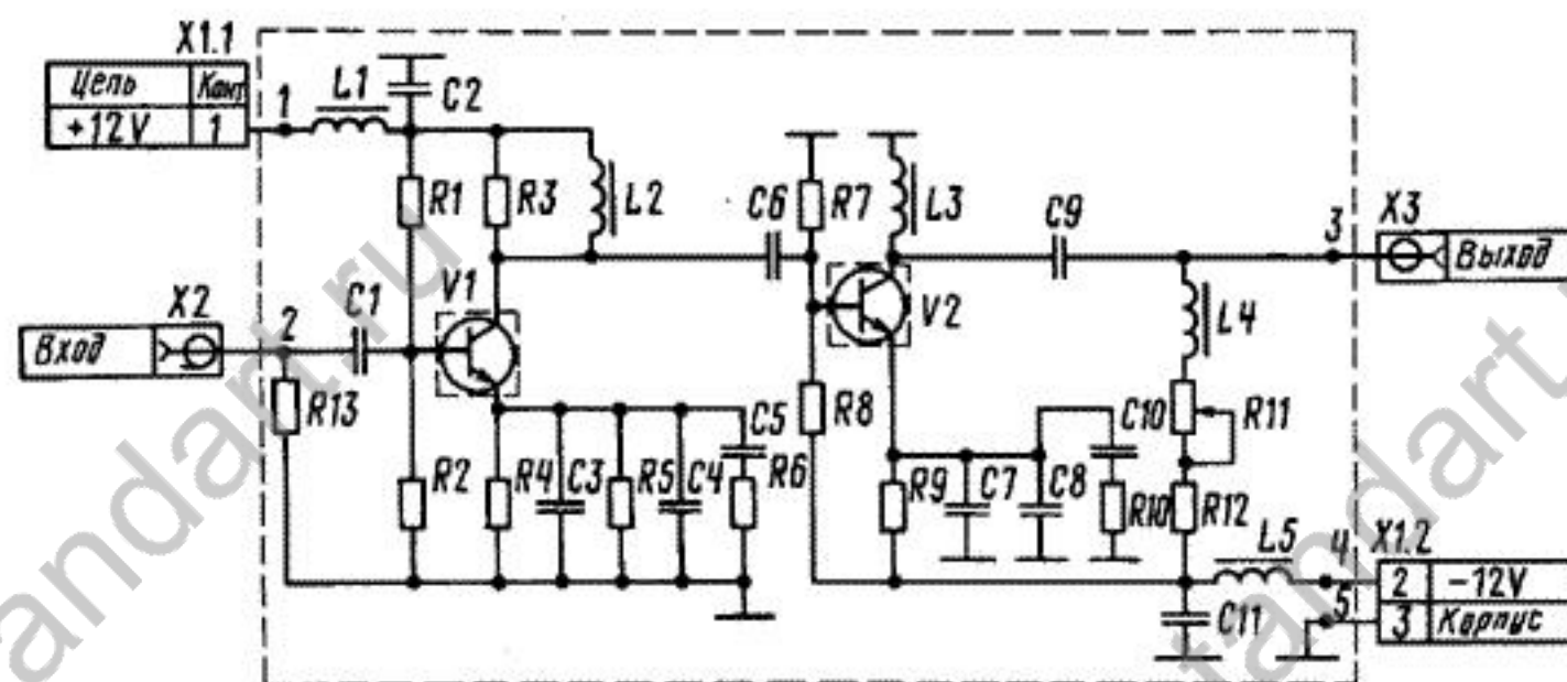
Рис. 2. Схема электрическая принципиальная усилителя ВЧ 2.030.055
