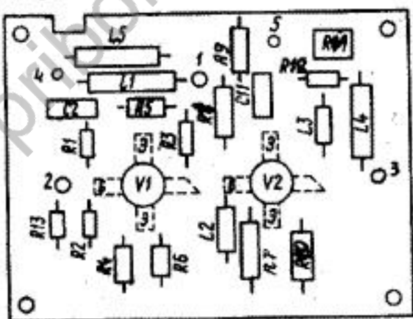
Рис. 3. Усилитель ВЧ 2.030.066
