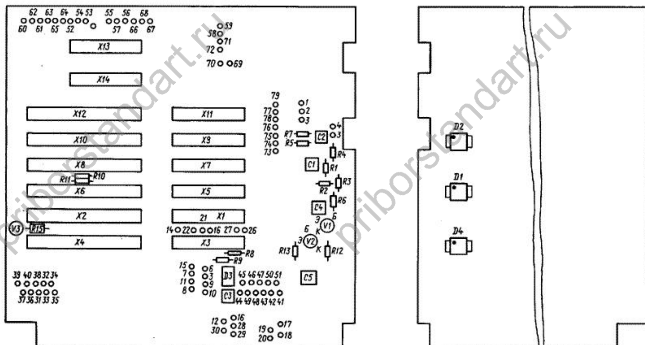
Рис. 20. Частотомер 5.171.007
