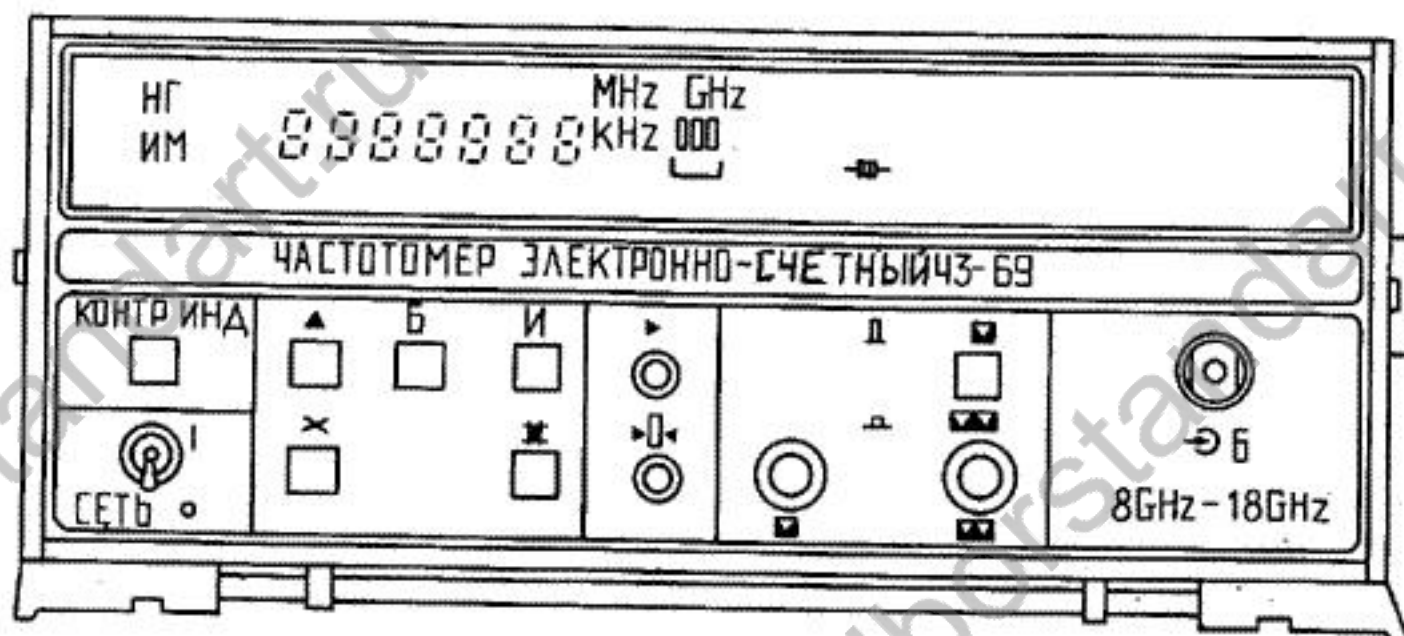
Рис. 2. Частотомер ЧЗ-69
