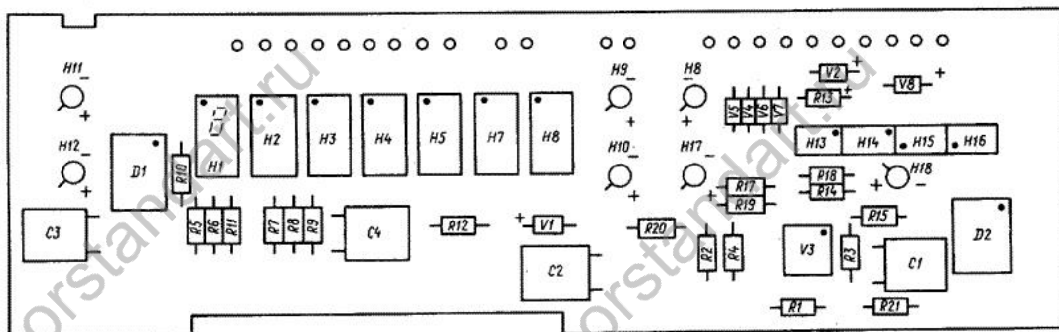
Рис. 10. Блок индикации 3.045.034
