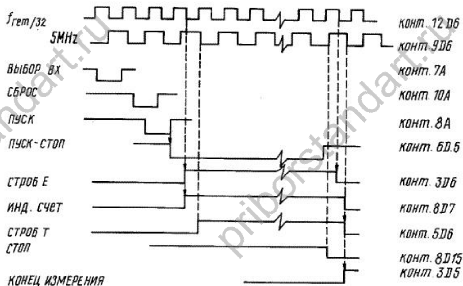
Рис. 5. Элюры напряжений работы счетчиков
