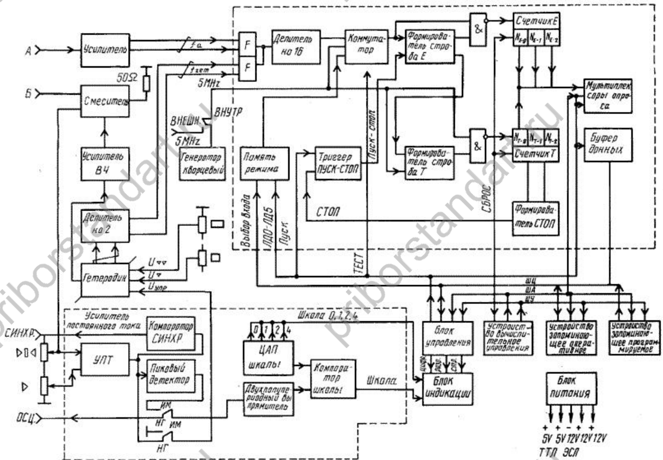
Рис. 4. Структурная схема приборов
