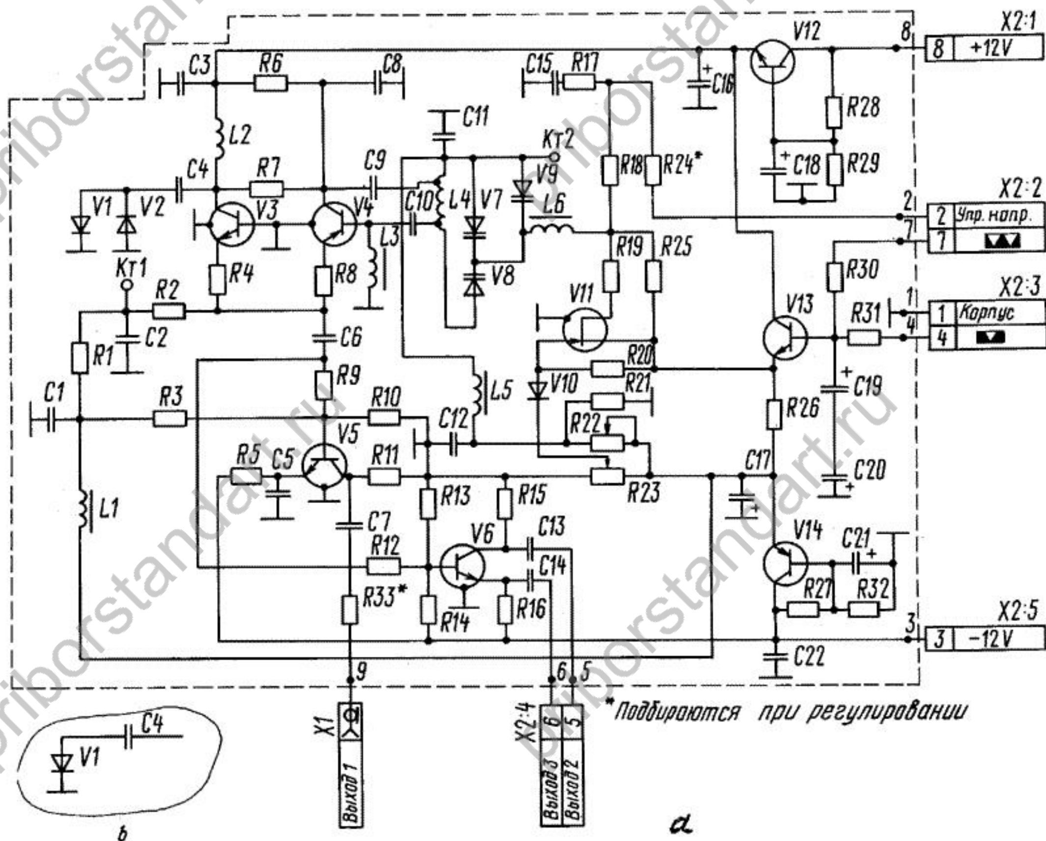
Рис. 4. Схема электрическая принципиальная гетеродина: а — 2.205.017; б — 2.205.017-01
