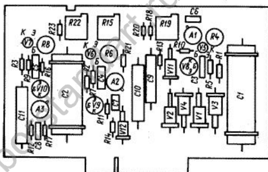
Рис. 17. Блок стабилизаторов напряжения 3.233.110
