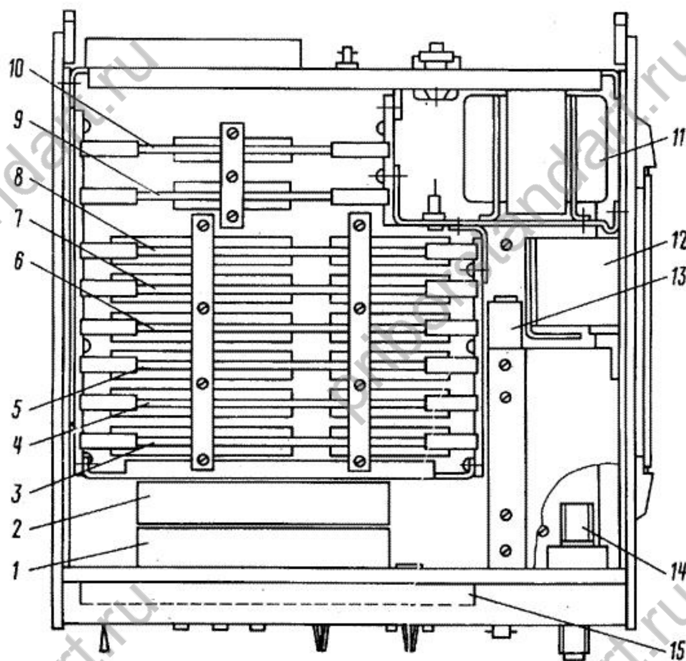
Рис. 1. Размещение основных составных частей:
