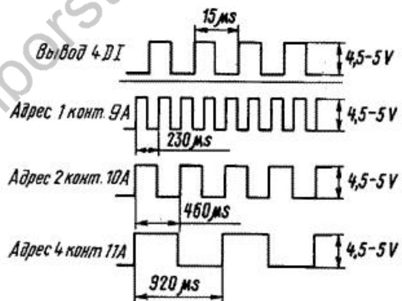
Блок управления 3.057.093
