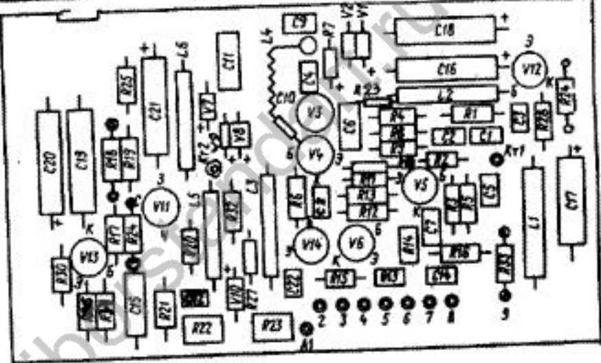
Рис. 6. Гетеродин 2.206.017
