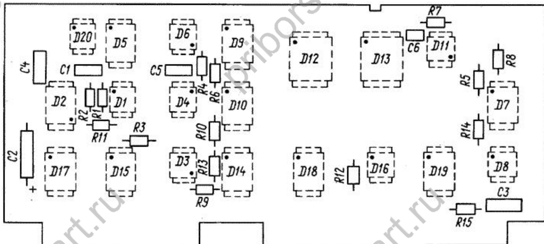
Рис. 13. Блок управления 3.057.093
