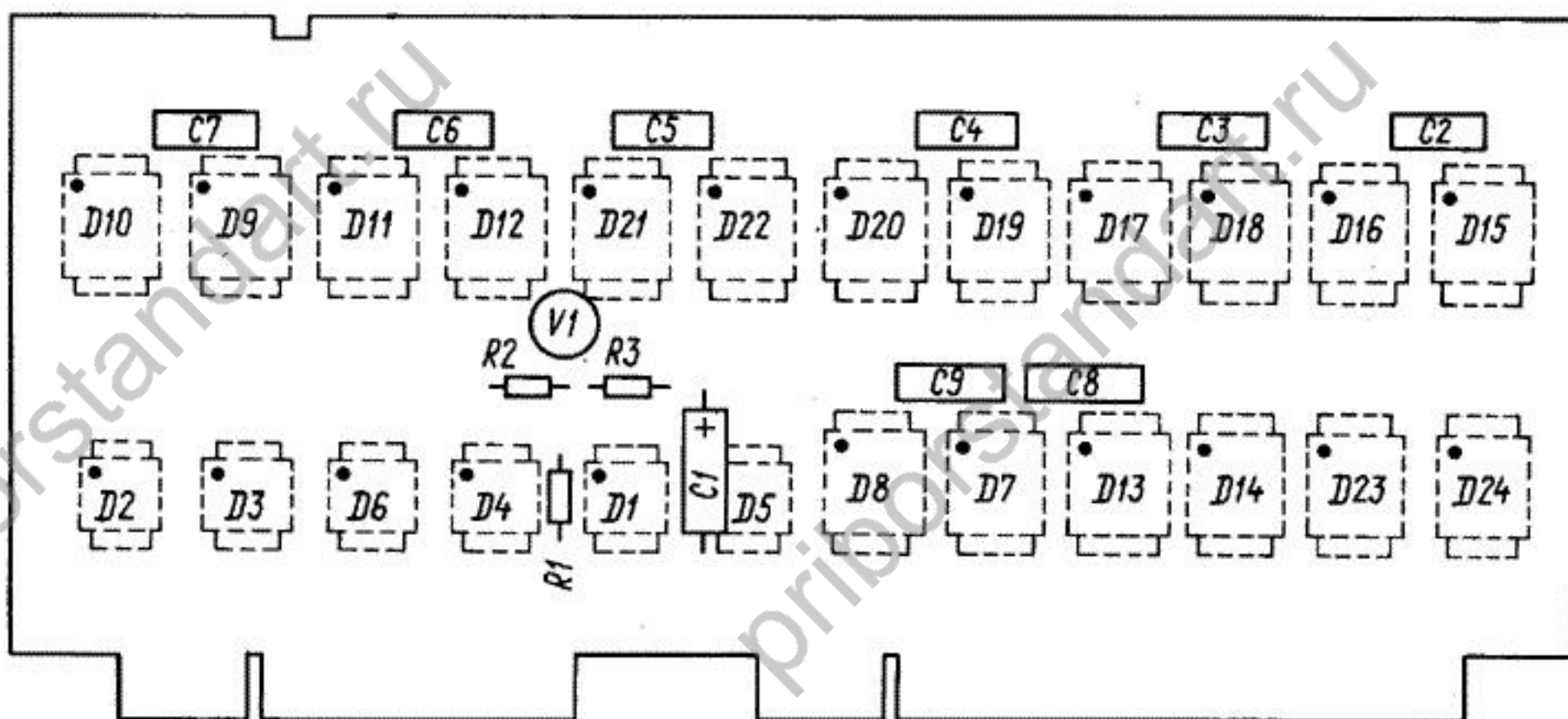
Рис. 16. Устройство запоминающее оперативное 3.065.067
