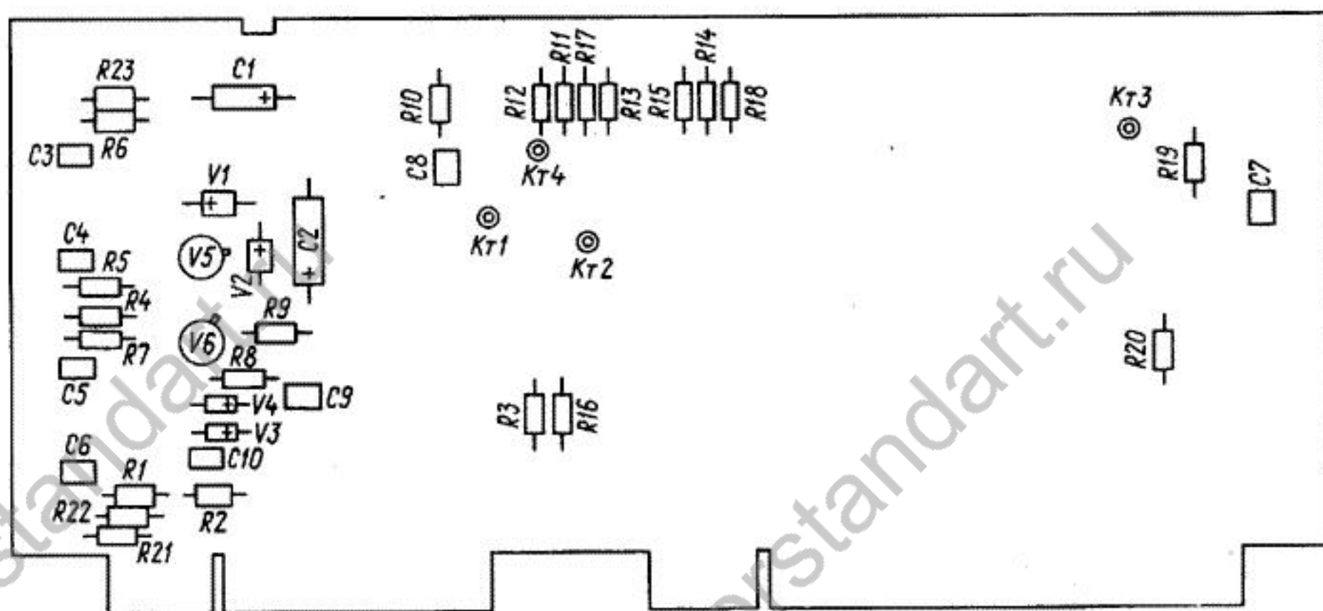
Рис. 11. Счетчик 3.056.034 (вид со стороны)
