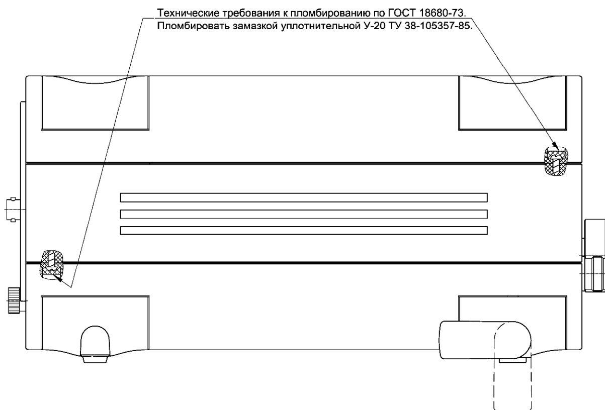
Рисунок 2. Места пломбирования и нанесения поверительных клейм
