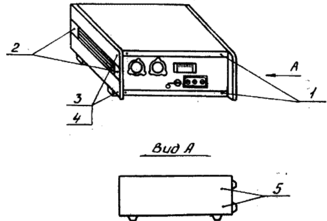
Рис. 10. Расположение крепежных винтов
