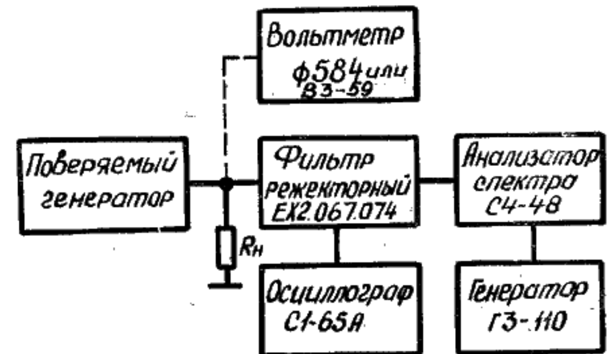
Рис. 8. Схема электрическая структурная подключения приборов для измерения коэффициента гармоник на частотах 10 и 20 кГц: R_n = (600 \pm 6) Ом; P \geq 0,2 Вт
