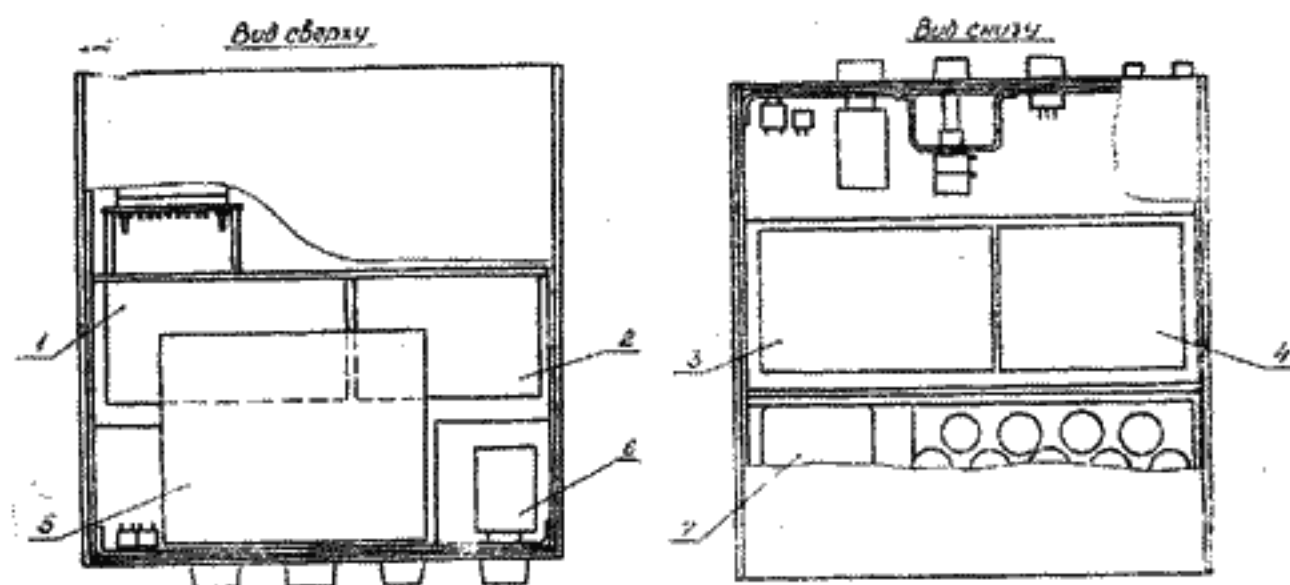
Рис. 11. Расположение узлов генератора
