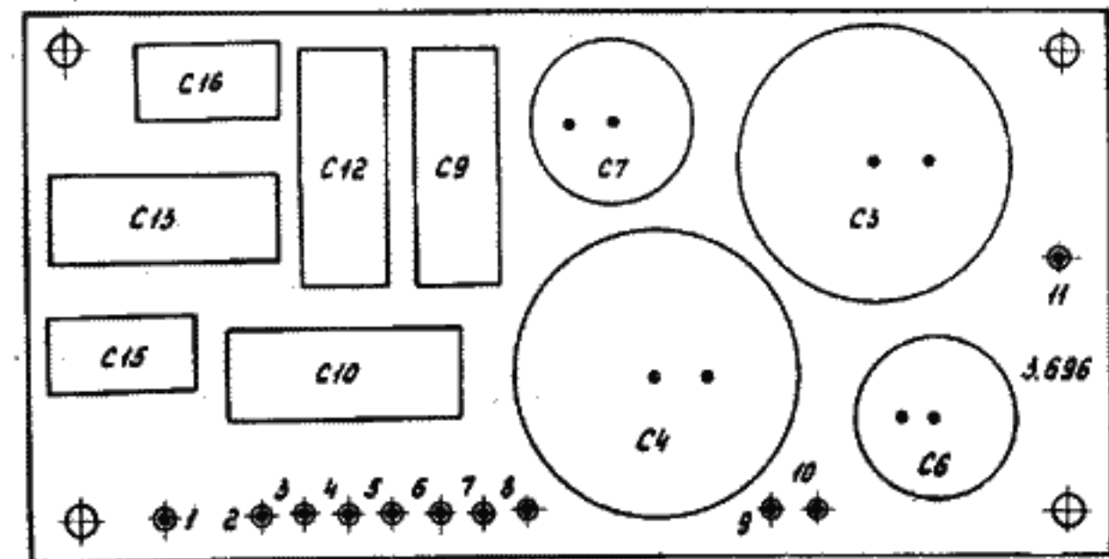
Рис. 10. Схема расположения электрических элементов платы фильтра режекторного 3.696
