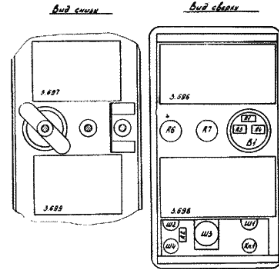
Рис. 9. Схема расположения электрических элементов фильтра режекторного
