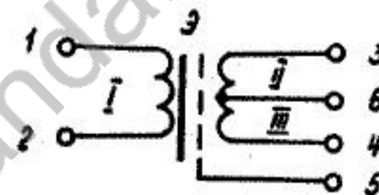
СХЕМА И ДАННЫЕ ОБМОТОК ТРАНСФОРМАТОРА
