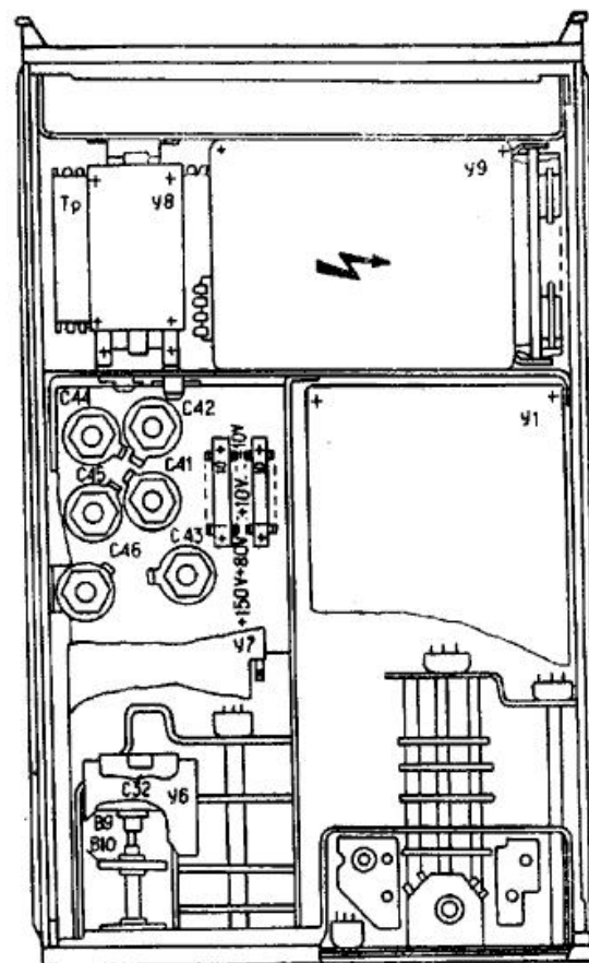
Рис. 4. Схема расположения установочных элементов и печатных плат (вид снизу)
