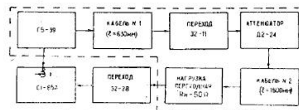
Рис. 7. Схема соединения приборов при определении времени нарастания переходной характеристики
