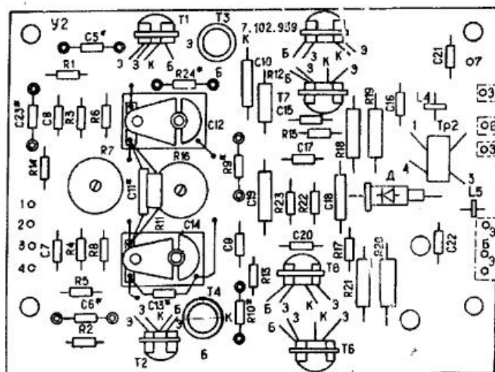
Рис. 2. Плата 6.673.326 СБ (Y2)
