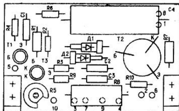
Рис. 9. Плата 6.673.478 СБ (У9-1)
