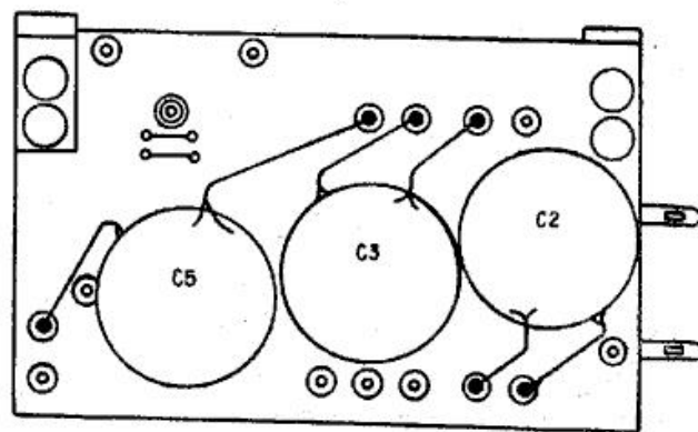
Рис. 11. Выпрямитель 5.087.063 СБ (V9-3)
