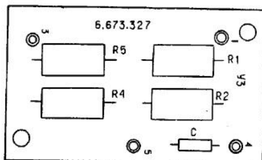
Рис. 3. Плата 6.673.327 СБ (Y5)
