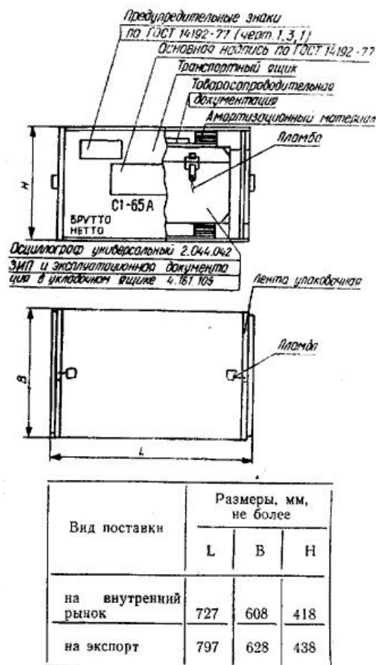
Рис. 11. Схема упаковки и маркирования упаковки
