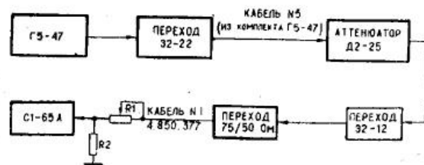
Рис. 10. Схема соединения приборов при определении неравномерности ПХ
