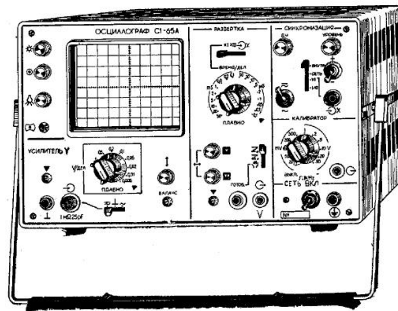
Рис. 1. Общий вид осциллографа
