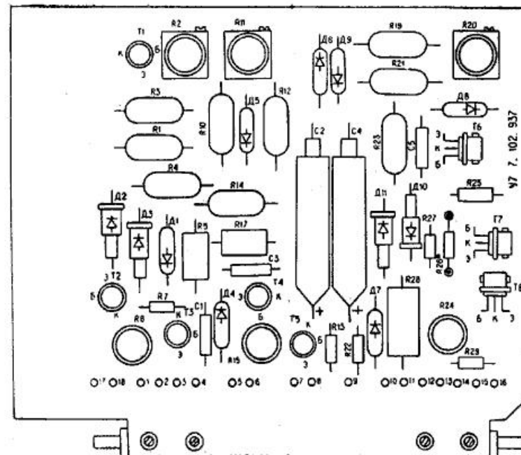
Рис. 7. Плата 6.673.323 СБ (У7)
