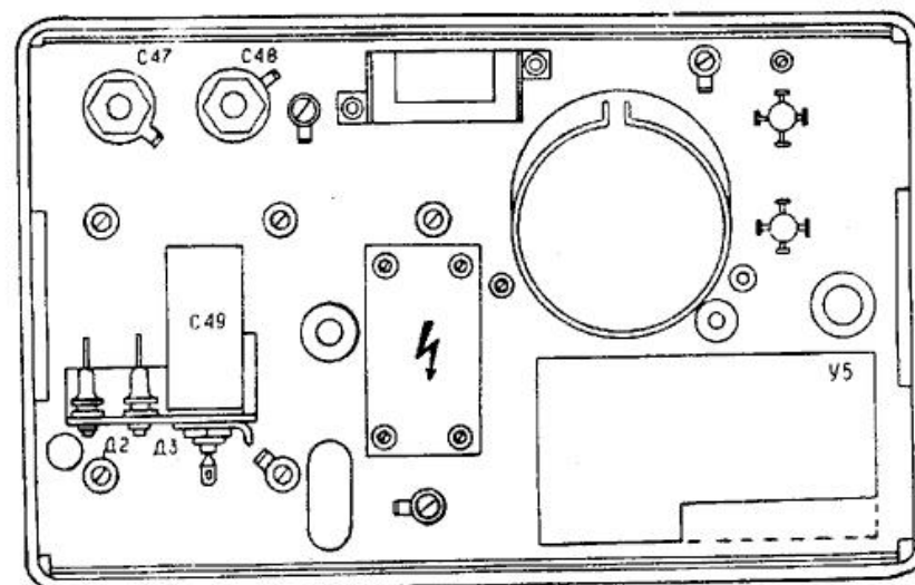
Рис. 6. Задняя стенка осциллографа. Расположение установочных элементов и печатных плат
