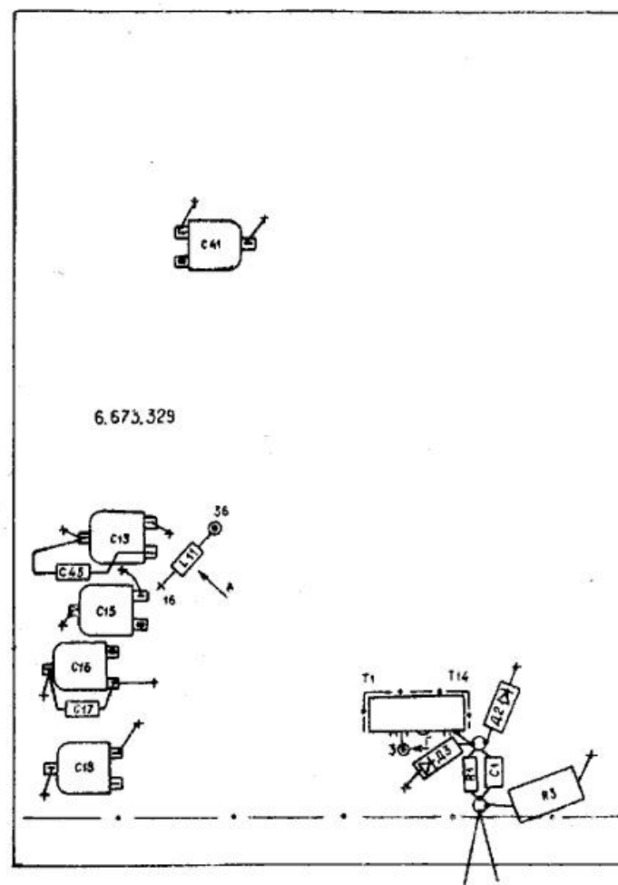
Рис. 1а. Плата 6.673.329 СБ (У1)
