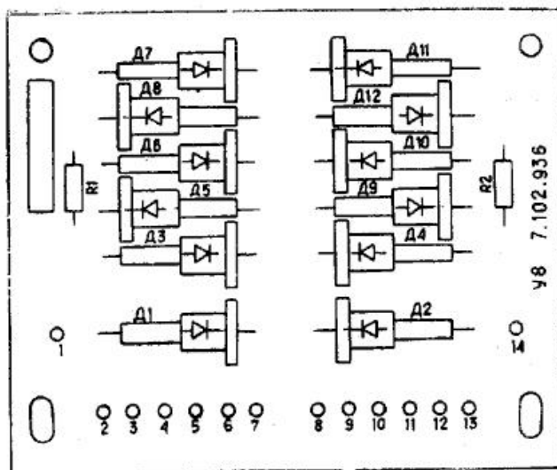
Рис. 8. Плата 6.673.322 СБ (У8)
