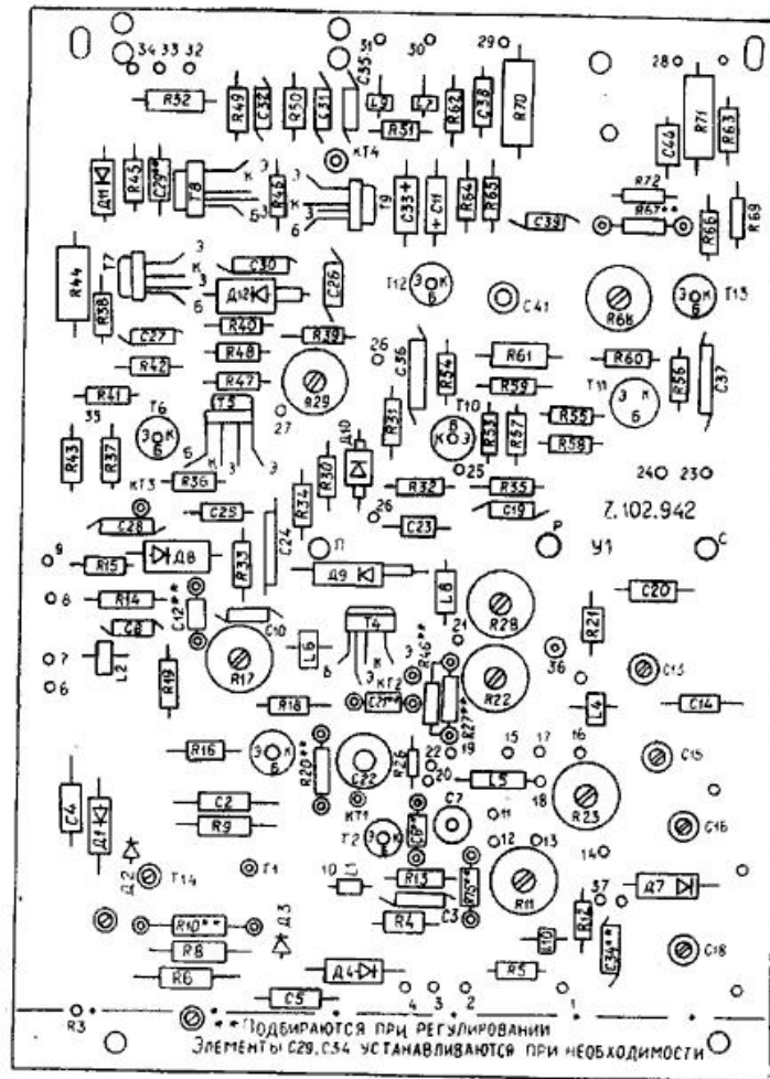
Рис. 1. Плата 6.673.329 СБ (У1)
