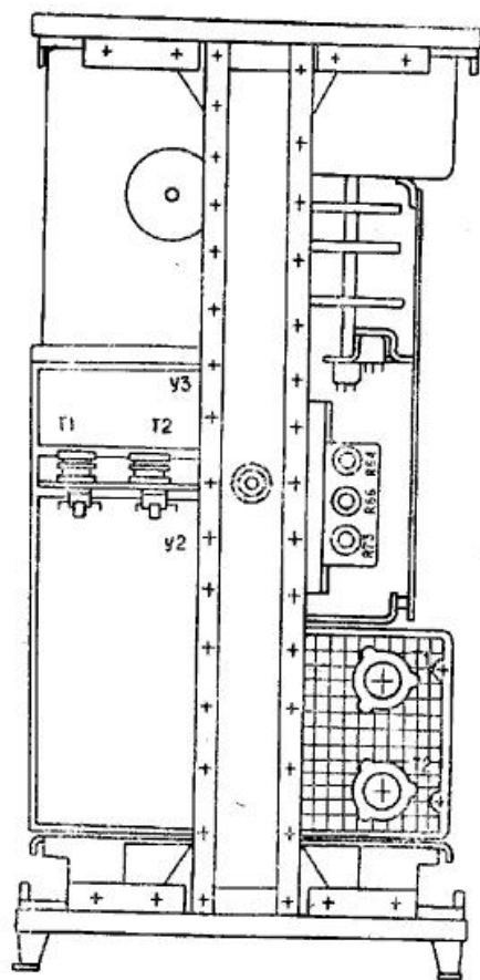
Рис. 5. Схема расположения установочных элементов (вид сбоку)
