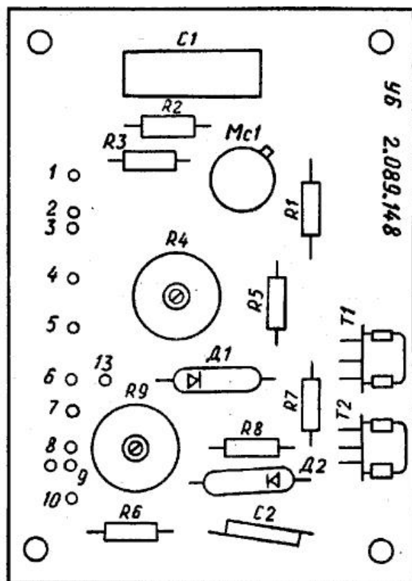
Рис. 6. Плата 2.089.148(У6)
