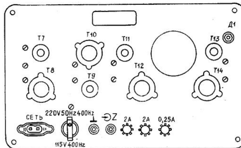
Рис. 7. Задняя стенка. Расположение установочных элементов
