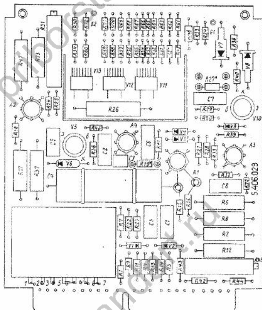
Преобразователь (пл. 5.406.029)
